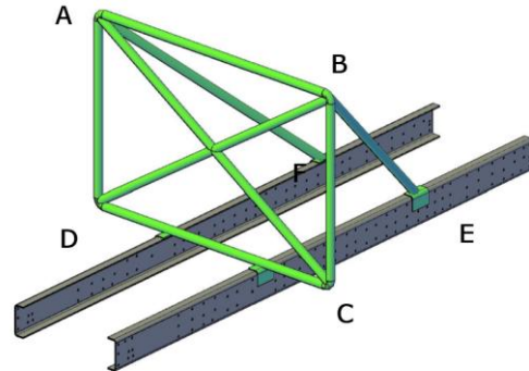
Dessin / Drawing 287-4
