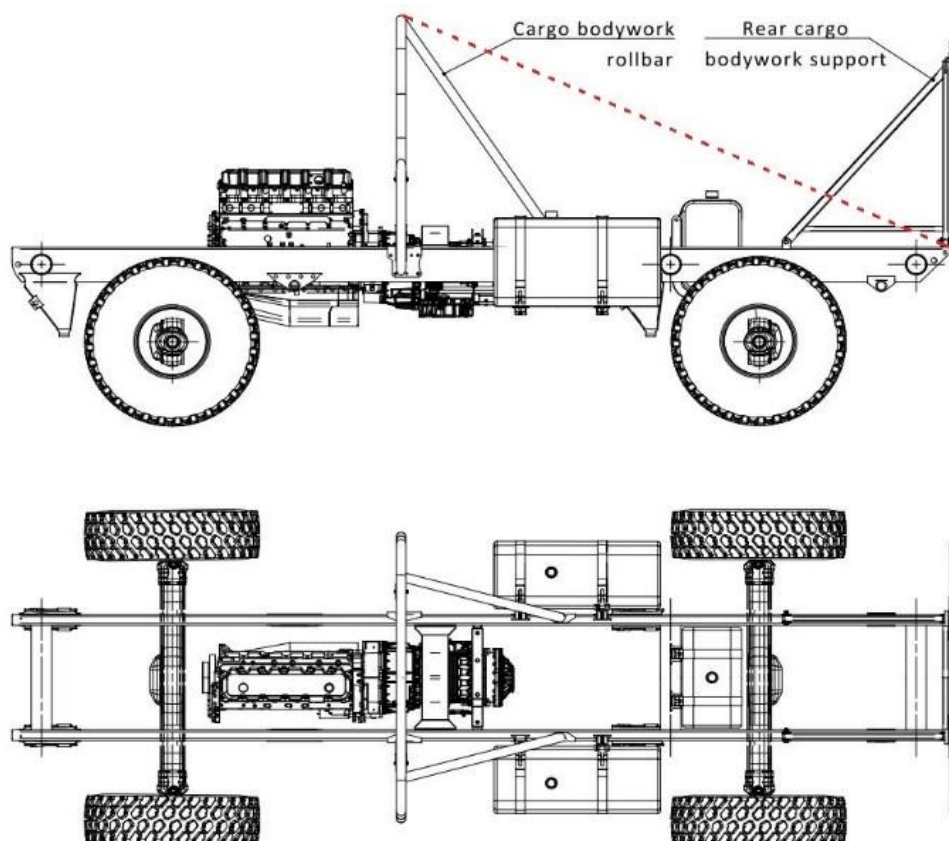
Dessin / Drawing 287-1
