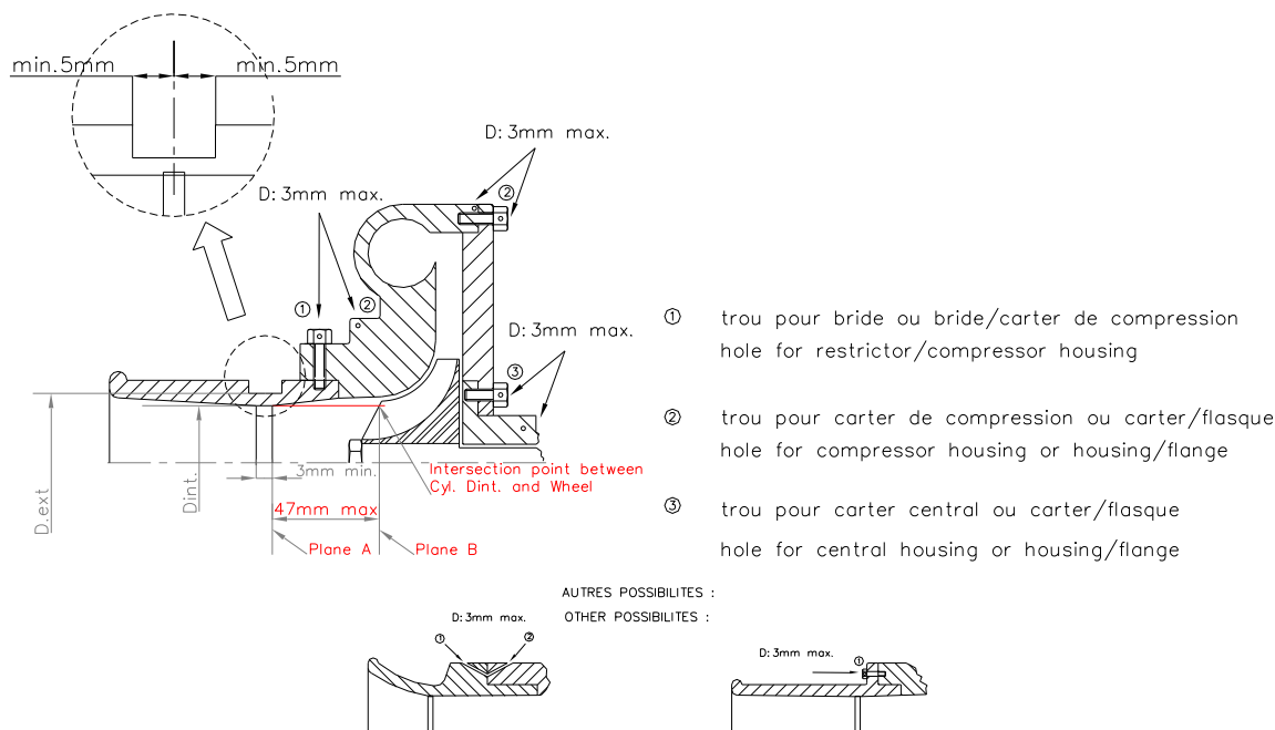
Dessin / Drawing 254-4
