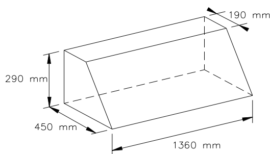
Dessin / Drawing 279-4
