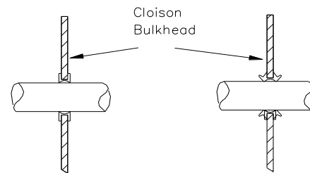
Dessin / Drawing 253-60
