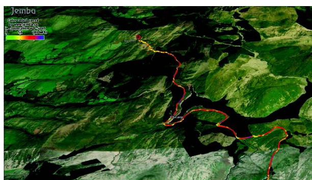
Trazado de velocidad antes de las recomendaciones
